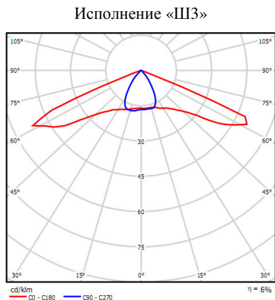
Рисунок 3 Кривые распределения силы света
