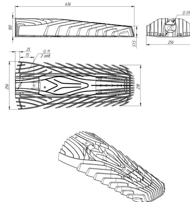
Рисунок 1 Габаритные размеры светильника « Superstreet»
