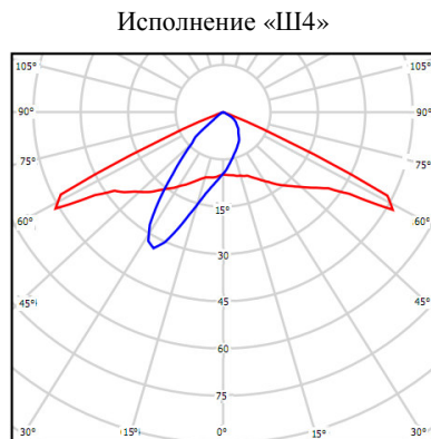
Рисунок 3 Кривые распределения силы света
